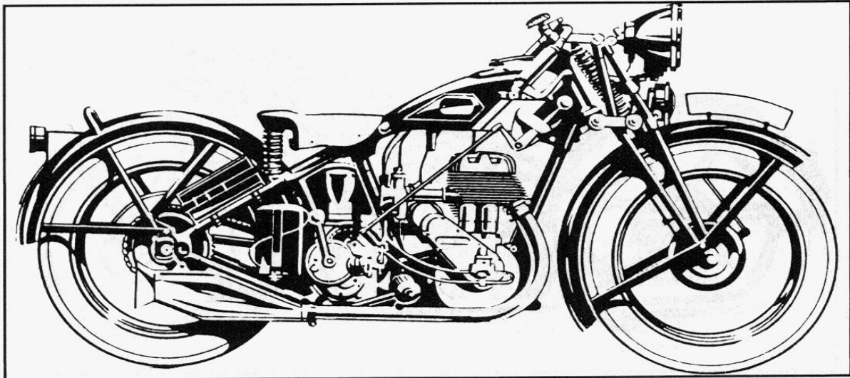
Deutsches „Kraft-Rad“: Modell „Universal“ mit 600er Columbus-Motor.
